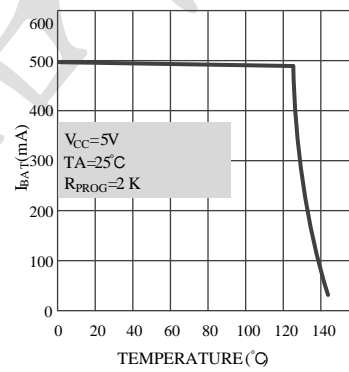
充电电流与芯片温度的关系曲线
