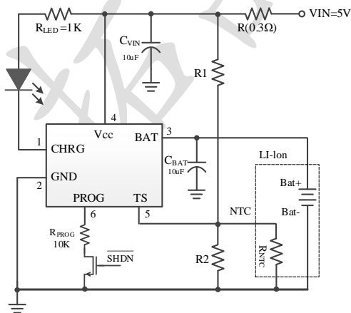
图 3 可信号控制充电电路
