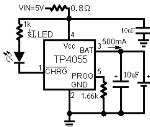
全功能单节锂电池充电器（接耗散电阻）
