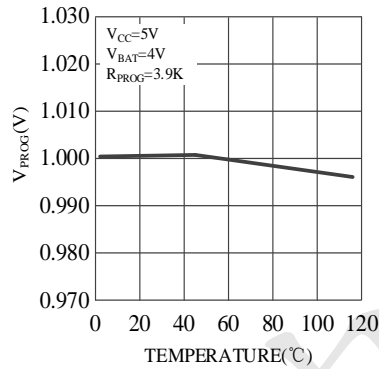
PROG 引脚电压与温度的关系曲线
