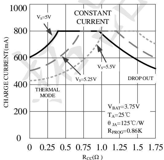
图 4: 充电电流与 RCC 的关系曲线
