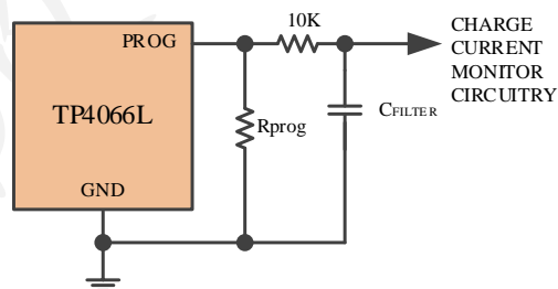
图 2：隔离 PROG 引脚上的容性负载和滤波电路 热考虑
