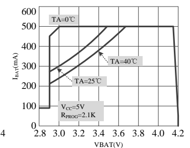
4.2V 充电电流与电池电压的关系曲线
