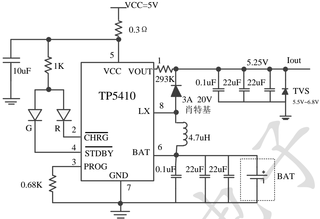
图 3 单节锂离子电池充电 1A 和微调升压 5.25V 输出控制器
