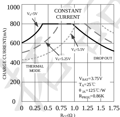
图 4：充电电流与 RCC 的关系曲线
