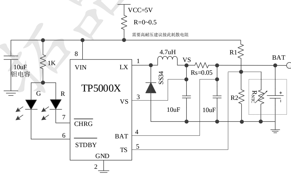
图 6 含温度检测的典型应用电路
